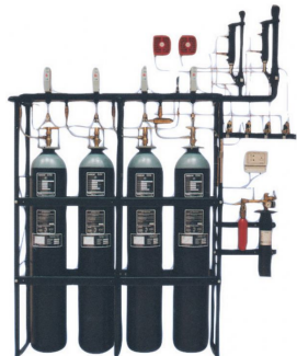
Bateria de 4 cilindres de CO2 de 67L
